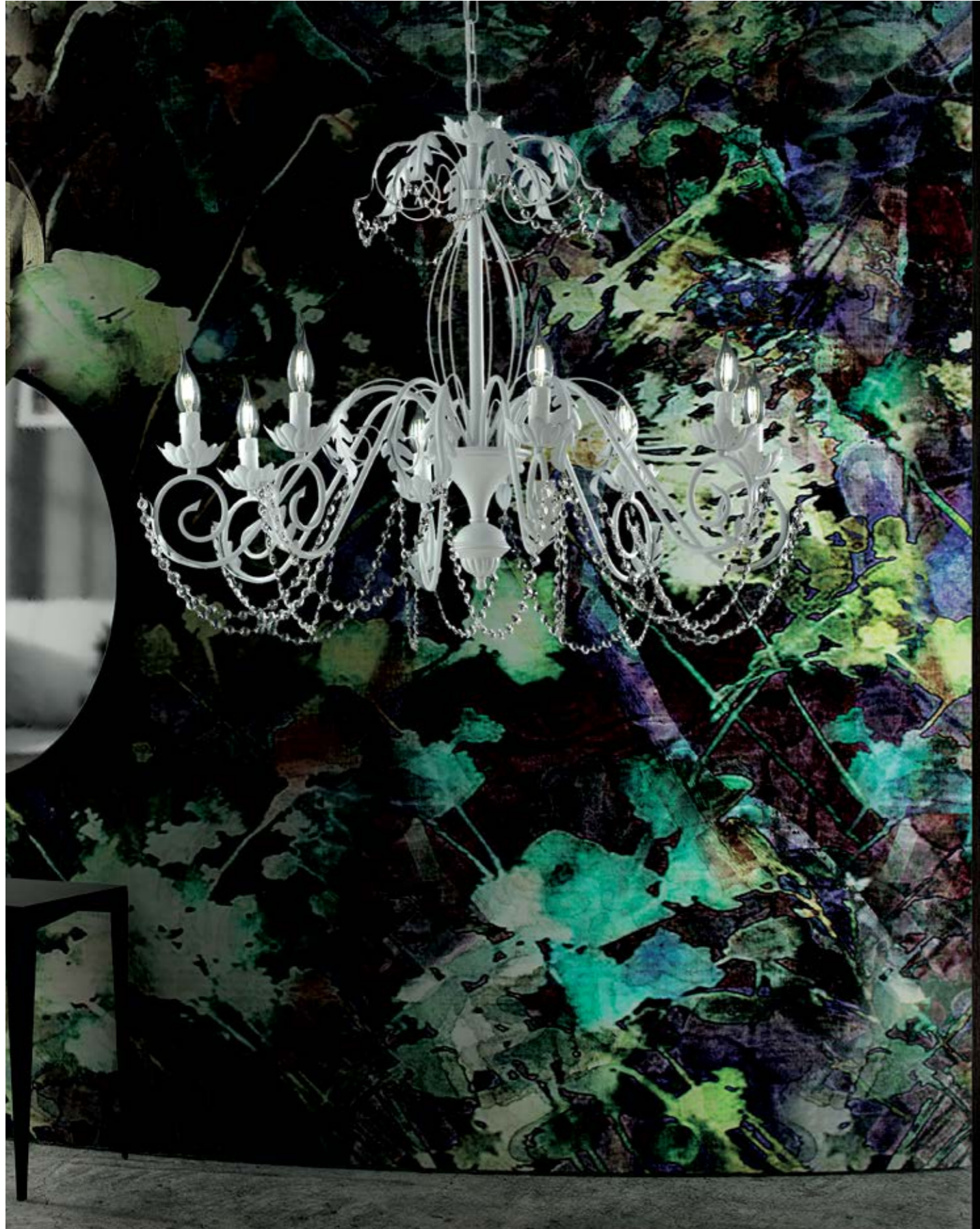
BL77-8-BCO H 70 Cm - Max 130 Cm Ø 90 Cm 8xE14 - 40 Watt Max
