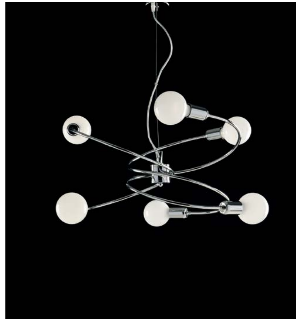
BL219-6-CR H 30 Cm - Max 130 Cm Ø 55 Cm 6xE27 - 60 Watt Max
