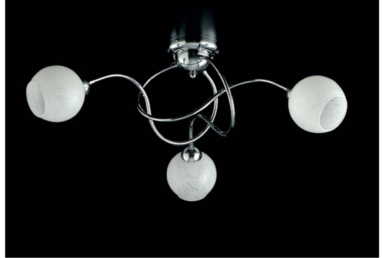
BL140-PL3-CR H 24 Cm Ø 60 Cm 3xE14 - 40 Watt Max
