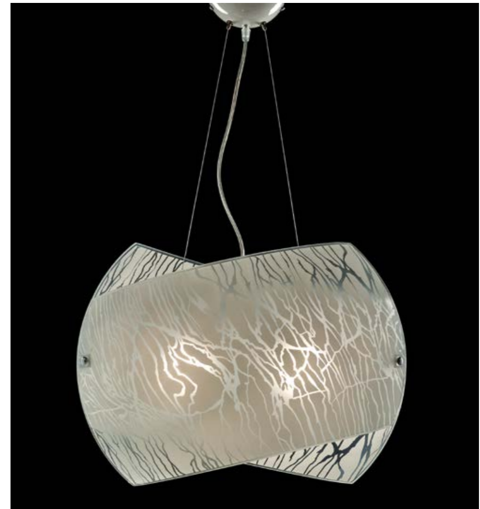
BL238-2-BCO H 40 Cm - Max 140 Cm Ø 52 Cm 2xE27 - 60 Watt Max
